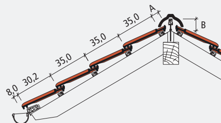
A = afstand van de bovenste panlat tot het snijpunt van de nok B = ruiiterhoogte
