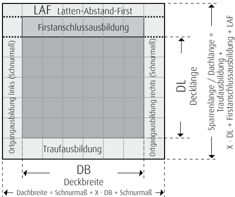
Ziegelaufbau
